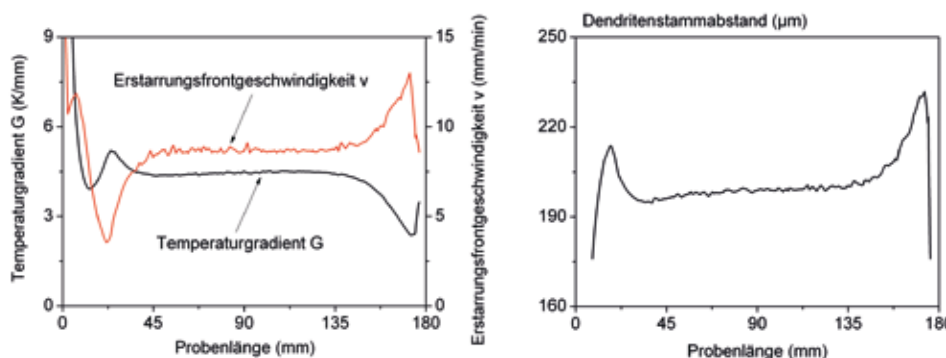
Berechnete Erstarrungsbedingungen (Temperaturgradient und Erstarrungsfrontgeschwindigkeit) und resultierender Dendritenstammabstand für eine gerichtet erstarrte Nickelbasislegierung.
