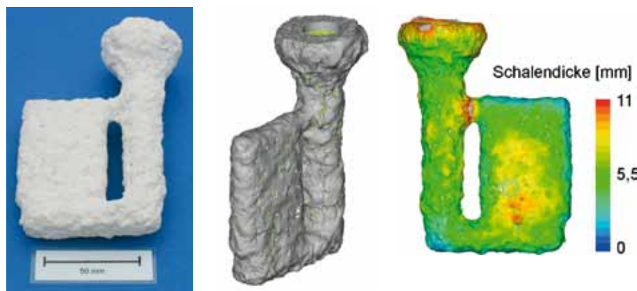
Reale und digitalisierte Formschalengeometrie im Vergleich: Durch die 3D-Vermessung von Formschalen mittels optischer Messsysteme kann ein exaktes Abbild der realen Formschale erzeugt werden. Die Schichtdickenverteilung ergibt sich durch die Vereinigung von Gusskörper und Formschale.
