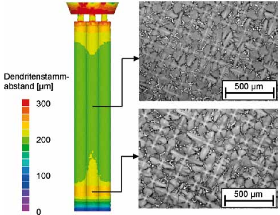
Berechnung und Experiment im Vergleich: Der rechnerisch ermittelte Dendritenstammabstand zeigt eine gute Übereinstimmung mit der experimentell festgestellten Mikrostruktur (DS).
